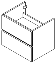
Unterschrank, 2x Schublade 57x50x43,5 cm DT060-XXXX
