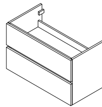
Unterschrank, 2x Schublade 82x50x43,5 cm DT085-3030 weiß glanz DT085-XXXX
