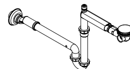
151.133.0 Siphon mit Klick-Klack Ablaufgarnitur, 32mm, Chrom (für Badmöbel-Waschtische)
